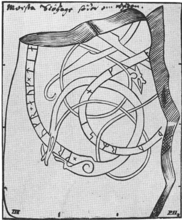
Fig. 188. U 191. Morsta, Össeby-Garns sn. Efter B 236.
